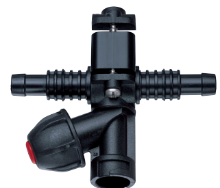
Schlauchanschluss doppelt Für Rohr-Außen-Ø 3/4" (25–28 mm O.D.) 065.275.56.KL.00 Für Rohr-Außen-Ø 1/2" (20–22 mm O.D.) 065.275.56.KH.00
